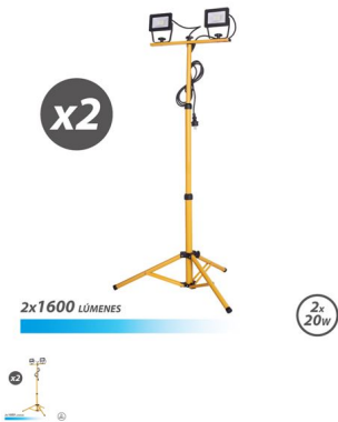
Foco LED Tripé 2x20W 1600 lumens Branco Frio 6500K ELBAT Cabo 3mts IP65 Uso Exterior
