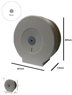
Suporte para Papel Higiénico Jumbo PW-5003
